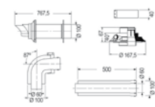
Kit salida realzada (boquilla + prolongador 0,5 m + codo 90° + terminal horizontal)
