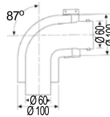
Codo 90°
