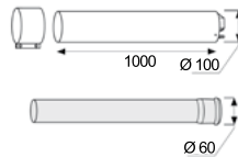
Prolongador 1 m
