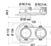
Separador de flujos
