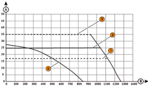
Curvas de la bomba de calefacción (muestran la relación entre presión y caudal)
