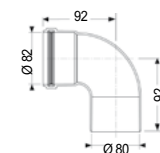
Codo 90° Ø 80
