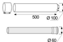
Prolongador 0,5 m
