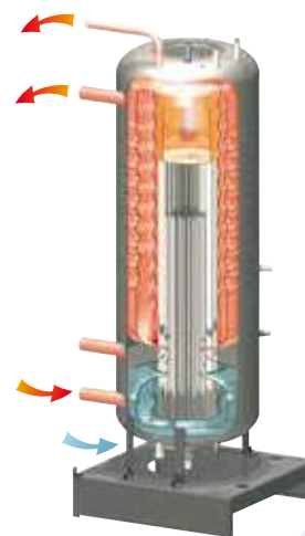
Detalle de funcionamiento de HM TC generando ACS y calefacción simultáneamente
